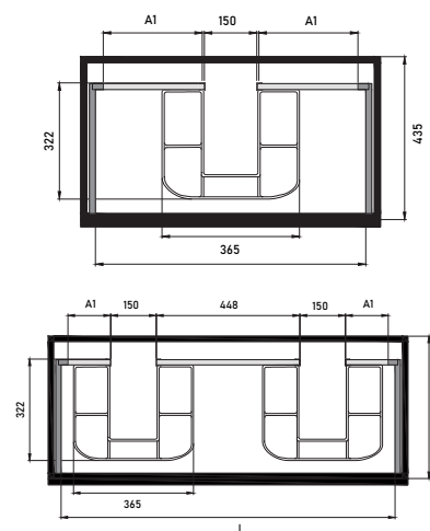
Cubrimiento antracita | Salvafón con separador / Anthracite Covering | Siphon Saver with Divider
