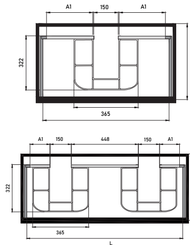
Cubrimiento antracita | Salvafifón con separador / Anthracite Covering | Siphon Saver with Divider
