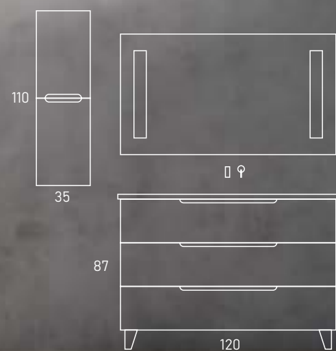
MODELO PARÍS Mueble 3 Cajones / 3-Drawer Unit | 120 x 45 x 87 cm Lacado en Verde Lago Mate / Matte Lake Green Lacquered Lavabo Encimera Cerámica / Countertop Ceramic Basin | 121 x 46 cm Blanco Brillo / Glossy White Semicolumna / Semi-column | 35 x 27 x 110 cm Lacado en Verde Lago Mate / Matte Lake Green Lacquered Espejo / Mirror | 120 x 80 cm Luz Integrada - LED / Integrated Light - LED
