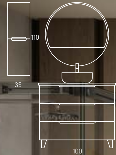
MODELO ROMA Mueble 3 Cajones / 3-Drawer Unit | 100 x 45 x 87 cm Lacado en Azul Egeo Mate / Matte Aegean Blue Lacquered Tapa Melamina / Melamine Top | 101 x 46 cm Desierto / Desert Lavabo Sobre Encimera / Countertop Basin Luisiana Blanco Brillo / Luisiana Glossy White Espejo / Mirror | 80 cm Ø Circular Luna/p Rayado Azul Egeo Mate / Circular Moon Scratch Matte Aegean Blue Semicolumna / Semi-column | 35 x 27 x 110 cm Lacado en Azul Egeo Mate / Matte Aegean Blue Lacquered
