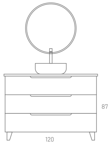
MODELO RUANDA Mueble 3 Cajones / 3-Drawer Unit | 120 x 45 x 87 cm Desierto/Negro / Desert/Black Tapa Melamina / Melamine Top | 121 x 46 cm Desierto / Desert Lavabo Sobre Encimera / Countertop Basin Luisiana Blanco Mate / Luisiana Matte White Espejo / Mirror | 80 cm Ø Eliot Round Luz Marco-LED / Eliot Round with Light Frame-LED
